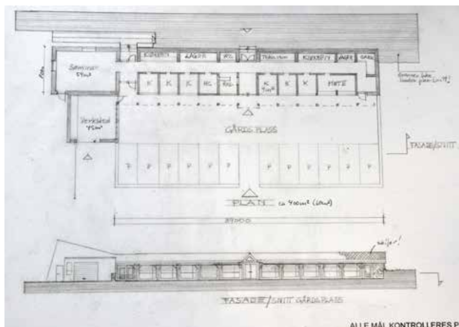
Skisse over nybygg for kontorer, servicebygg og forsamlingsrom.
